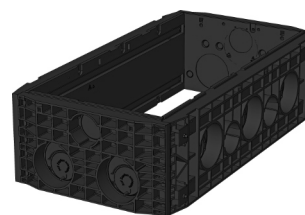
Rama 350 mm Nr produktu: BP-101489 3 x Ø 110 / 2 x Ø 160 / 36 x Ø 30 5 x Ø 110 / 3 x Ø 160 Waga: 53 kg
