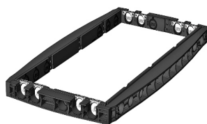
Rama 70 mm nakładana Nr produktu: na zapytanie 4 x nakładana / 1 x Ø 50 6 x Ø 50 Waga: 9,1 kg
