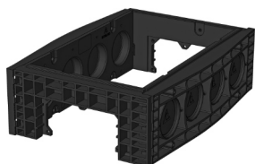
Rama 220 mm Nr produktu: BP-101850 1 x prostokąt 4 x Ø 110 Waga: 12,5 kg
