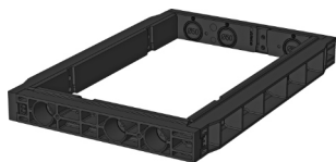
Rama 70 mm Nr produktu: BP-101847 3 x Ø 50 3 x Ø 50 Waga: 3,8 kg
