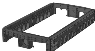
Rama 220 mm Nr produktu: BP-103636 1 x Ø 110 / 2 x prostokąt 8 x Ø 110 Waga: 49,0 kg
