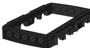
Rama 220 mm Nr produktu: BP-102699 5 x Ø 110 4 x prostokąt Waga: 39,0 kg
