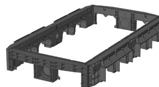
Rama 220 mm Nr produktu: na zapytanie 1 x Ø 110 / 2 x prostokąt 4 x prostokąt Waga: 46,0 kg
