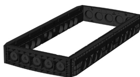
Rama 220 mm Nr produktu: BP-102757 5 x Ø 110 9 x Ø 110 Waga: 55,0 kg
