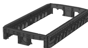
Rama 220 mm Nr produktu: BP-104544 2 x prostokąt / 1 x Ø 110 9 x Ø 110 Waga: 50,0 kg
