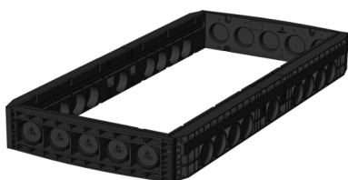
Rama 220 mm Nr produktu: BP-102784 5 x Ø 110 12 x Ø 110 Waga: 67,0 kg
